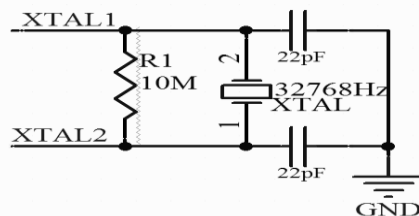
外部晶振电路参考
