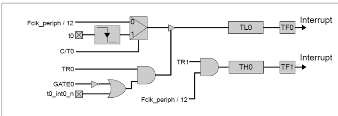
Timer0/1-mode3
