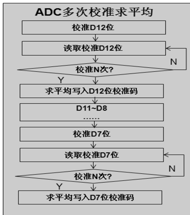
ADC多次校准求平均
