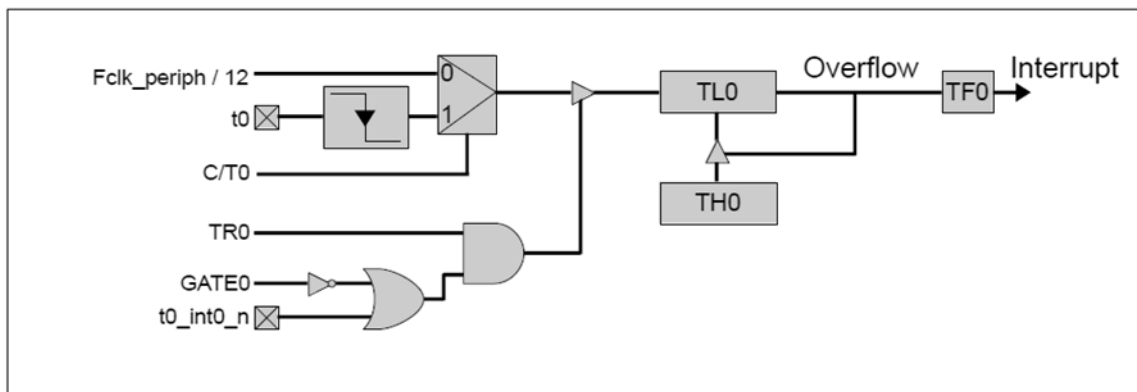
Timer0/1-Mode2
