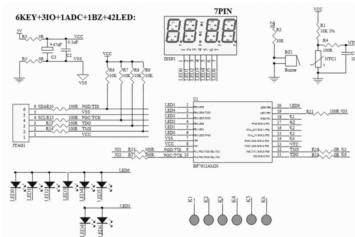
BF7612AM20 参考电路
