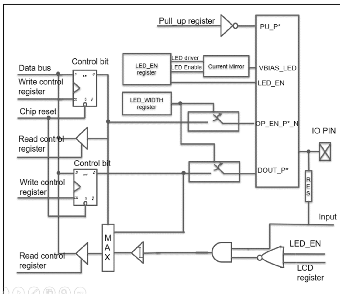
LED 结构图
