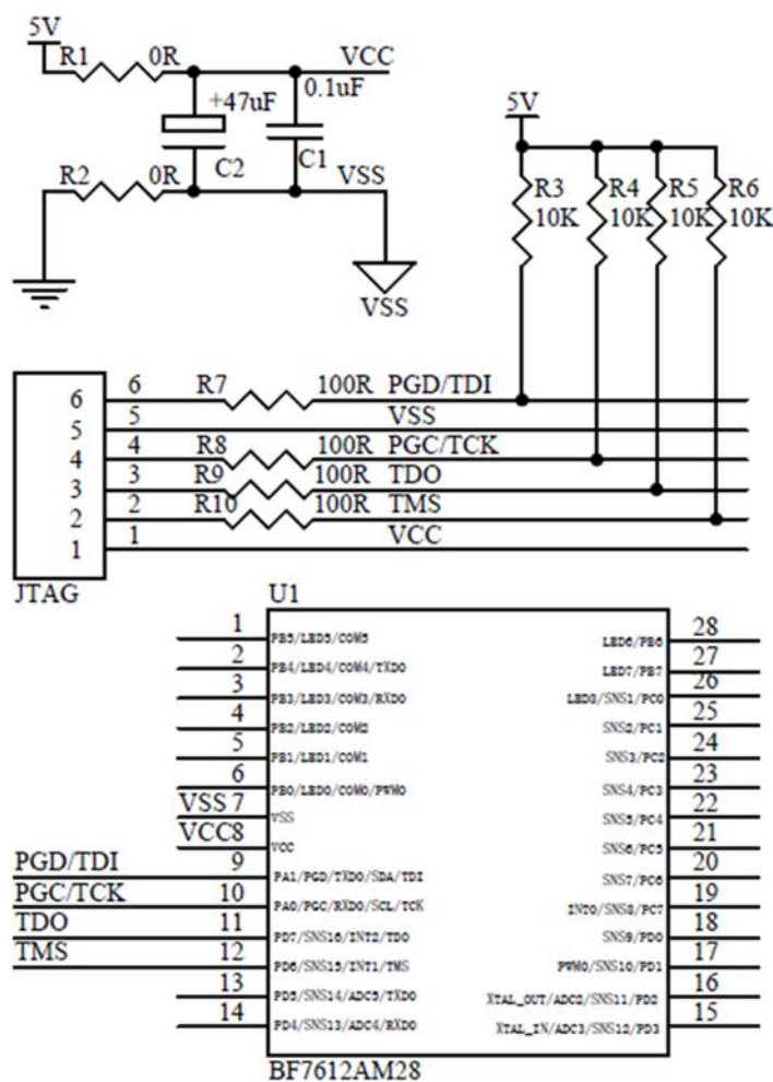
JTAG 连接示意图
