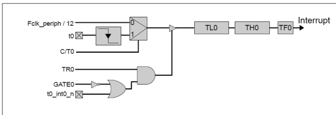
Timer0/1-Model
