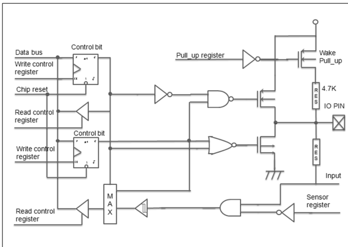
帶 Sensor 功能的 IO 结构
