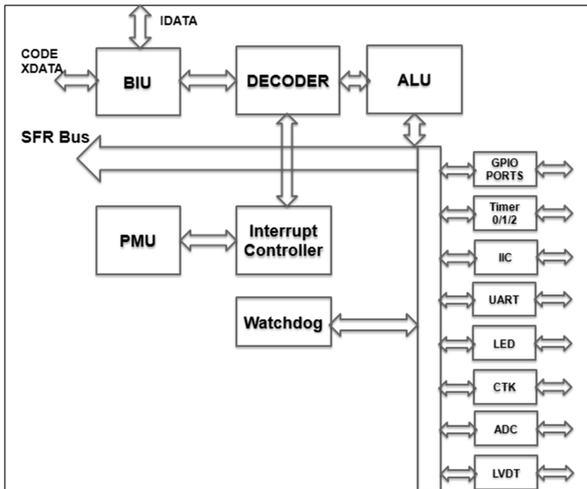
系统总线
