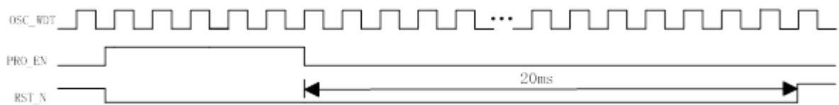
编程复位
