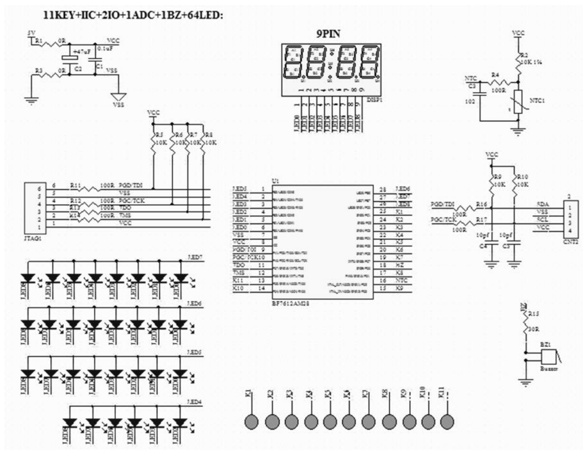
BF7612AM28 参考电路
