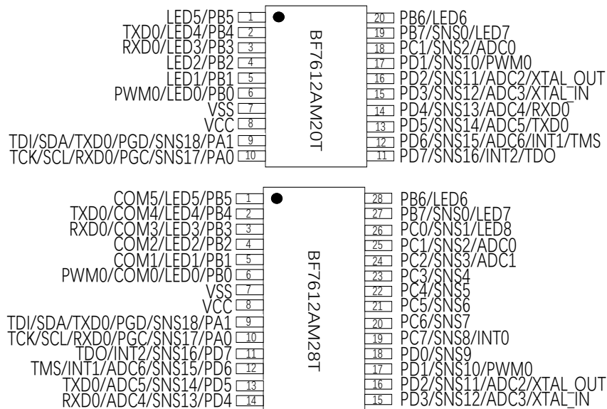
引脚配置
