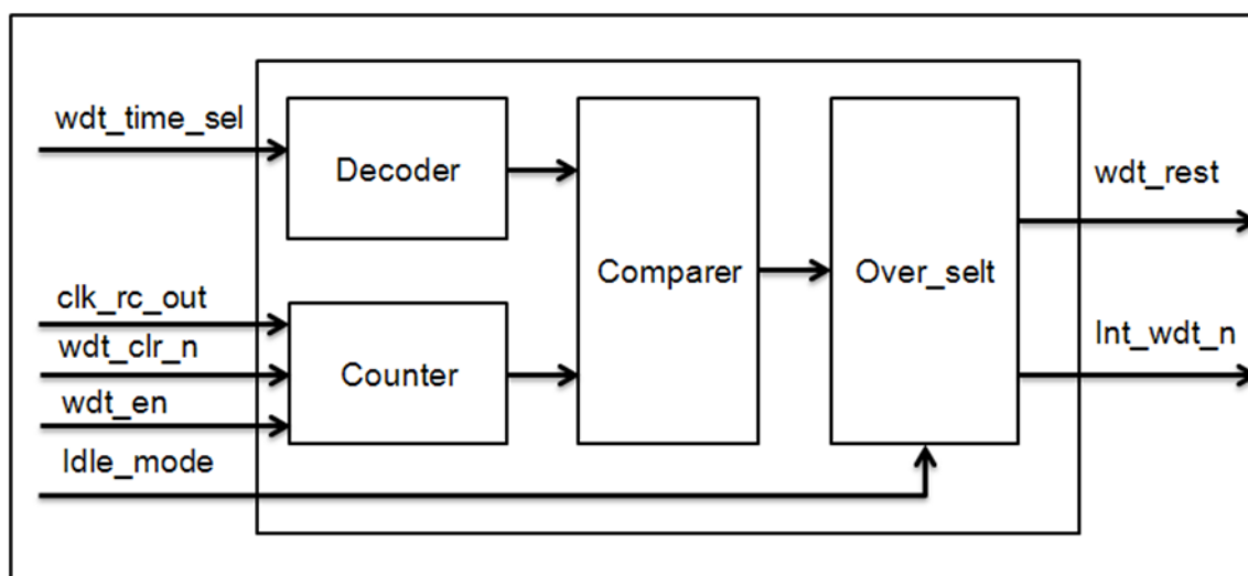
WDT 框图
