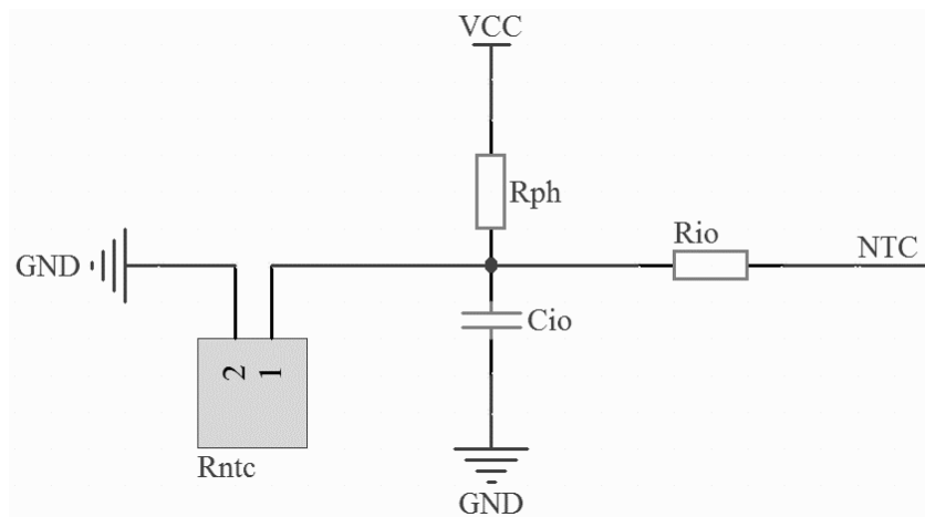
温度检测参考电路
