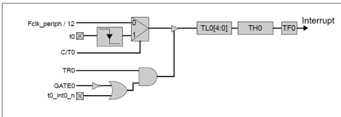
Timer0/1-Mode0
