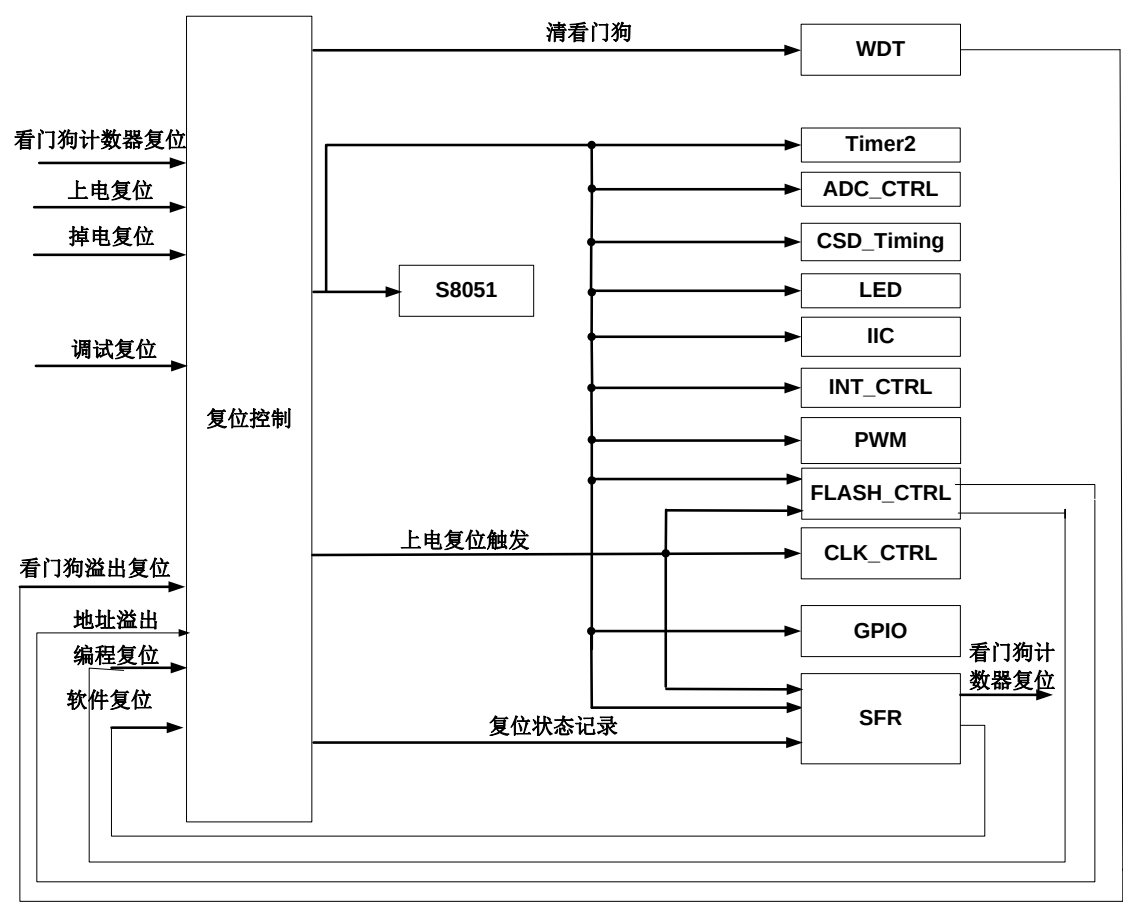
复位方框图
