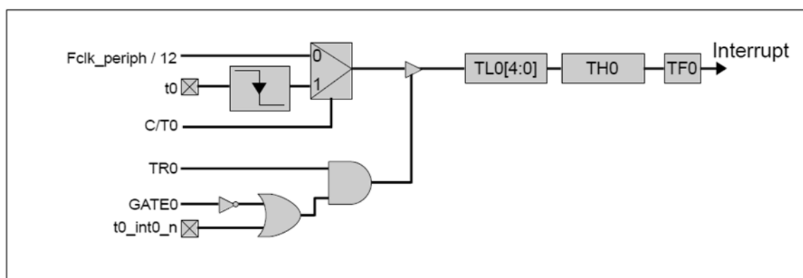
模式 0 逻辑逻辑结构图
