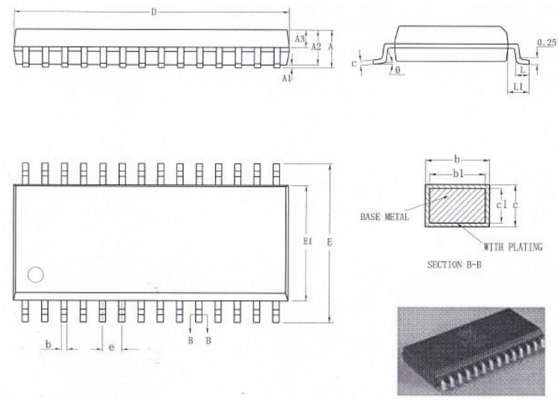
SOP28 封装信息图
