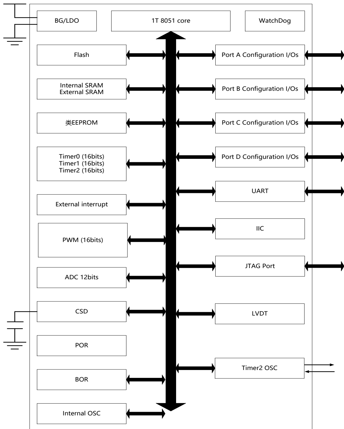
系统框图
