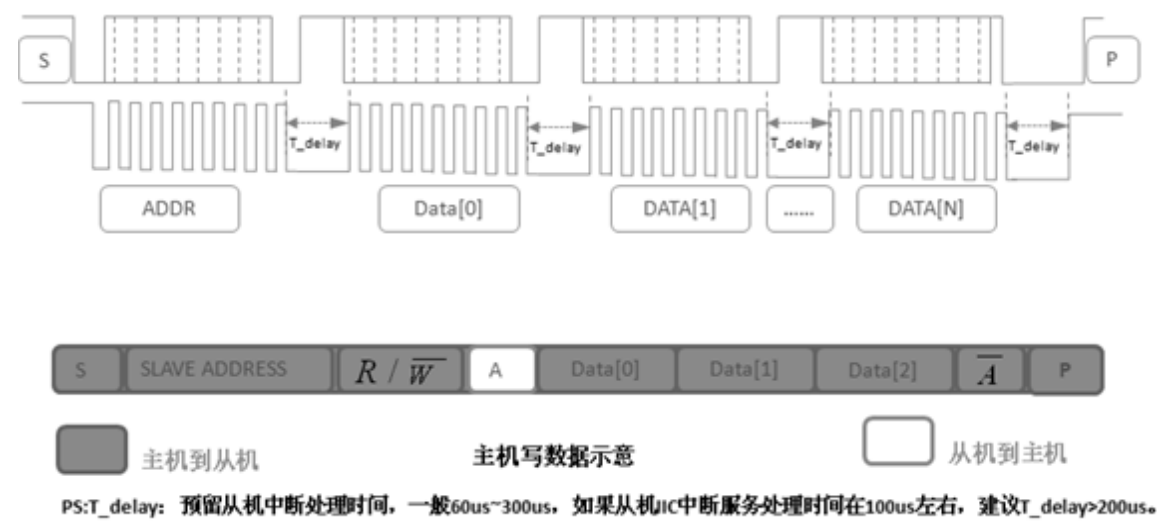
IIC 主机写数据示意图
