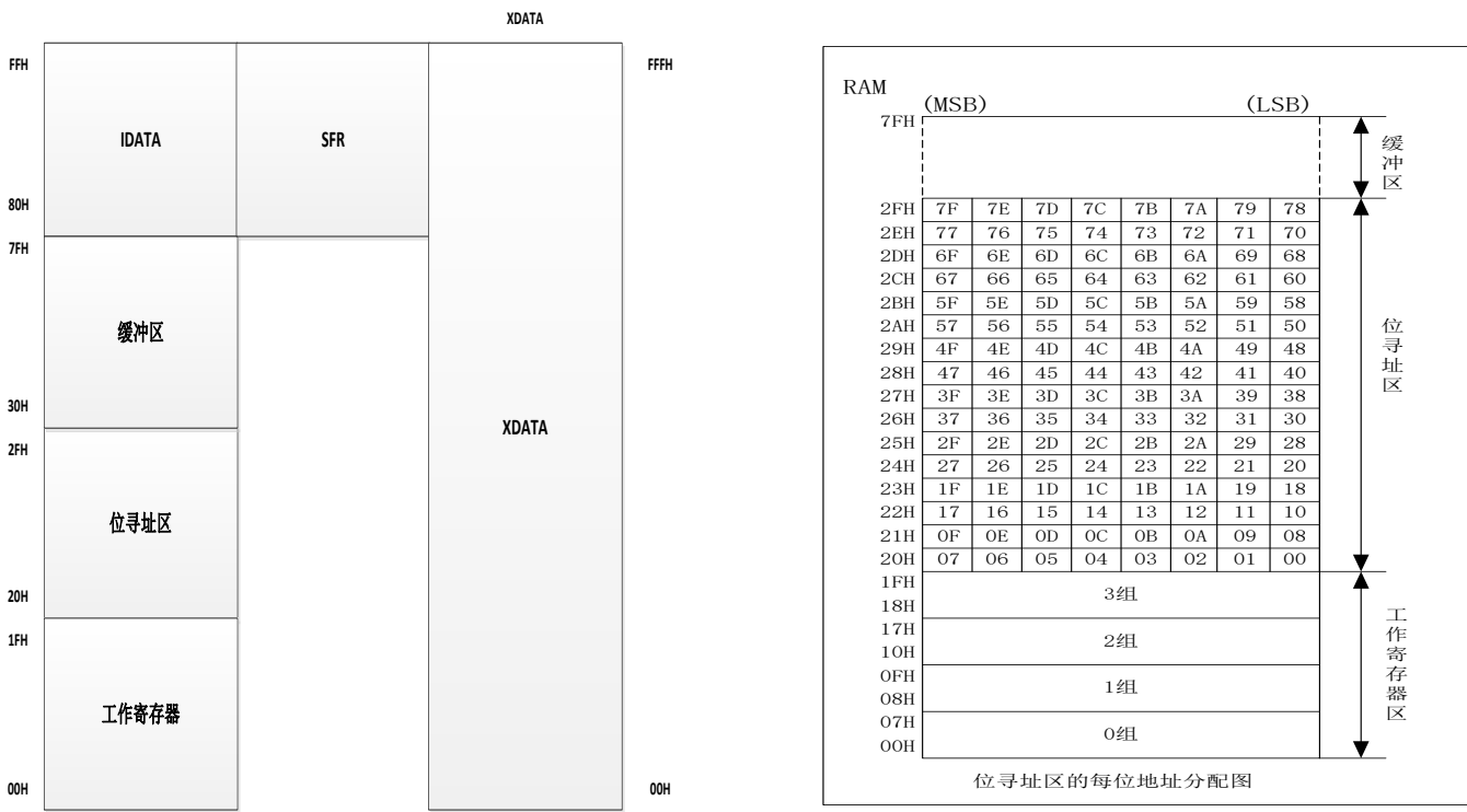
RAM 地址空间分配图
