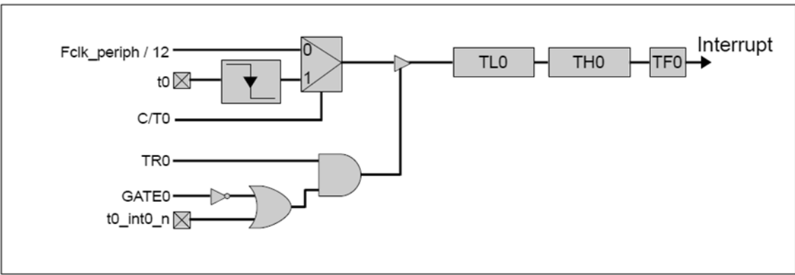
模式 1 逻辑逻辑结构图
