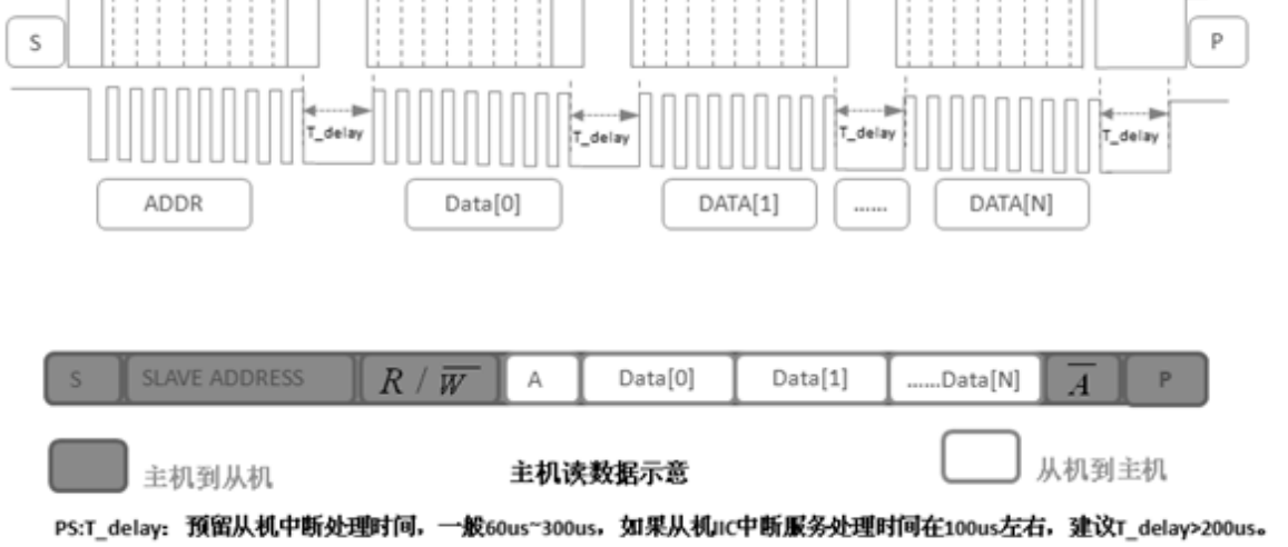
IIC 主机读数据示意图
